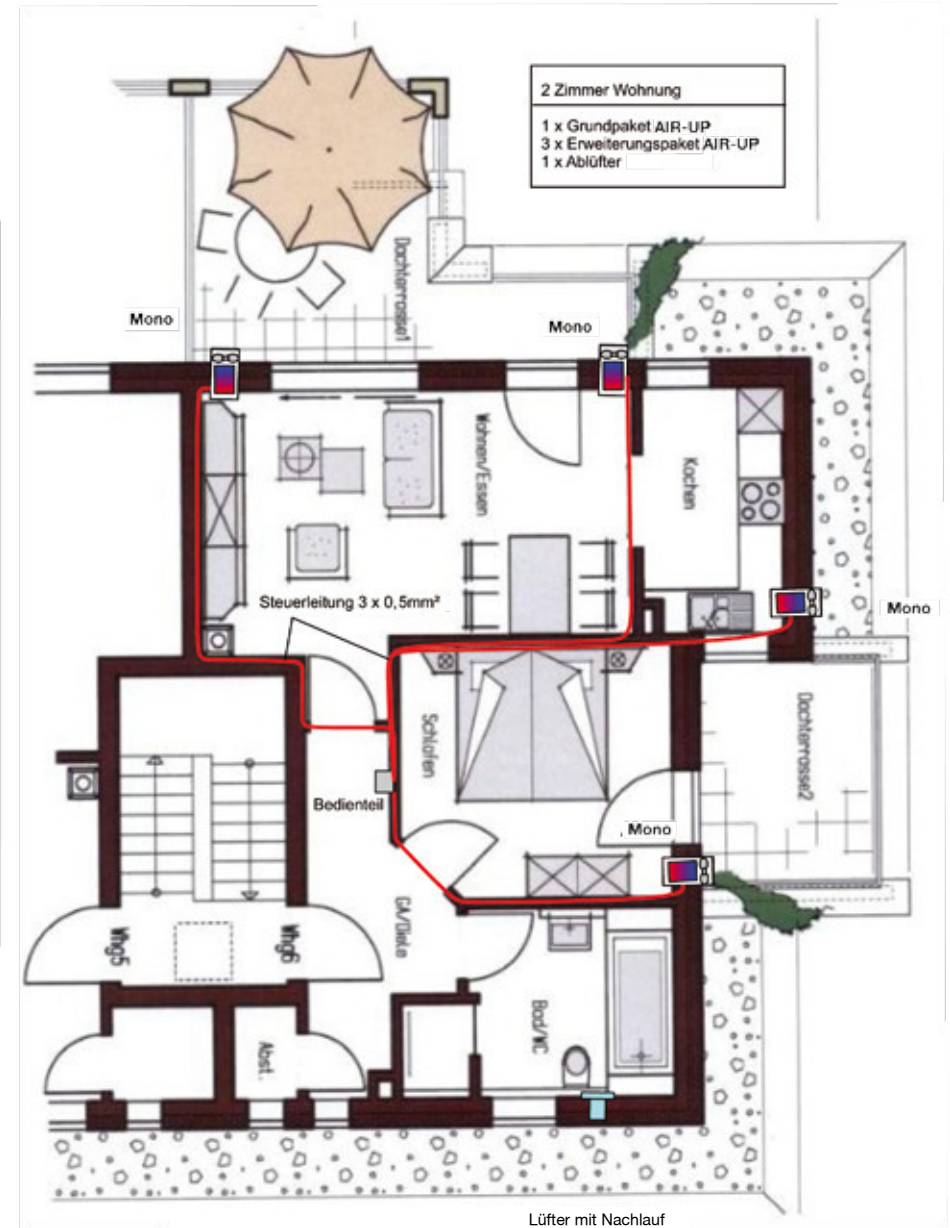
Lüfter mit Nachlauf und Feuchtesensor
